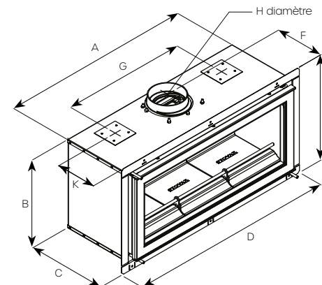
Dimensions Insert
